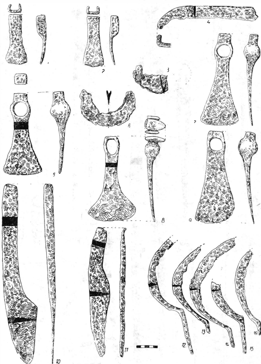
Fig. 2. — Dragostoveni. Unelte agricole. 1, 2, oticuri; 3, 6, rame de hirleț; 4, coasă; 5, 7—9, săpălīgi; 10, 11, cuțite de plug; 12—16, seceri.
