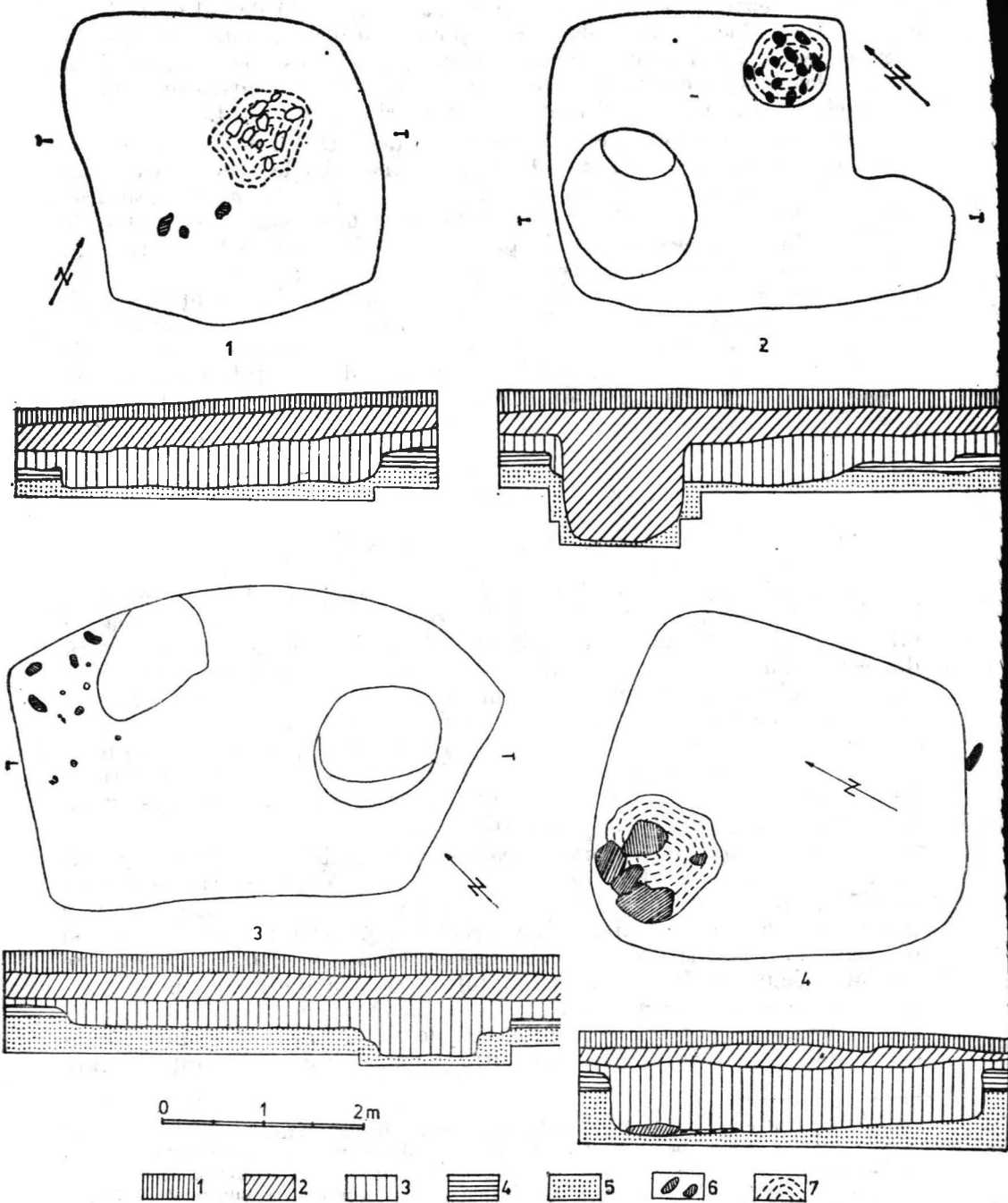
Fig. 2. Botoșana, jud. Suceava. Planul și profilul semiordeielor 1, 2, 3 4; 1 sol arabil; 2 nivel prefeudal; 3 nivel și locuințe adincite de epocă Latène; 4 strat de culoare brun închis; 5 sol viu; 6 pietre; 7 resturi de vatră.
