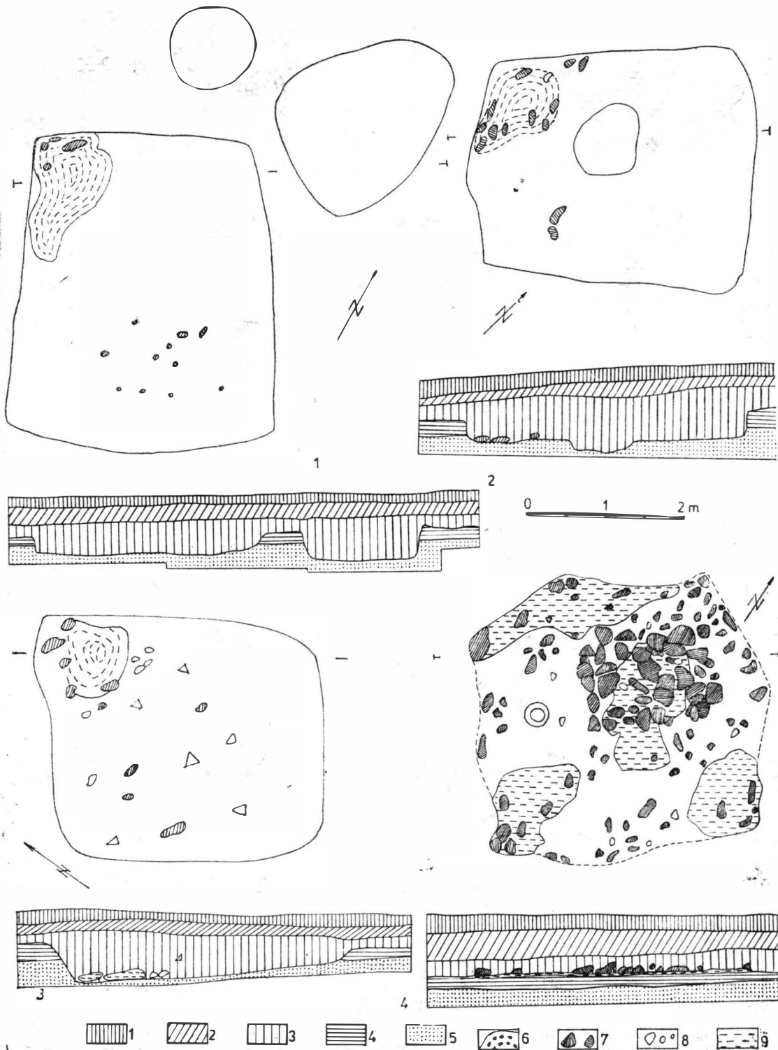
Fig. 5. Botoșana, jud. Suceava. Planul și profilul semiordeielor, 8, 10, 15 și ale locuinței de suprafață 1; 1 sol arabil; 2 nivel prefeudal; 3 nivel și locuințe de epocă Latene; 4 strat brun închis; 5 sol viu; 6 resturi de vatră; 7 pietre; 8 fragmente ceramice; 9 pământ ars cu resturi de chirpici.
