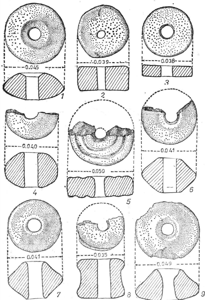
Fig. 13. Botoșana, jud. Suceava. Obiecte din lut ars; 1 locuința 3; 2 locuința 12; 3 semibordeiul 2; 4 locuința 2; 5 semibordeiul 4; 6 din stratul de cultură; 7 semibordeiul 1; 8 semibordeiul 8; 9 semibordeiul 5.
