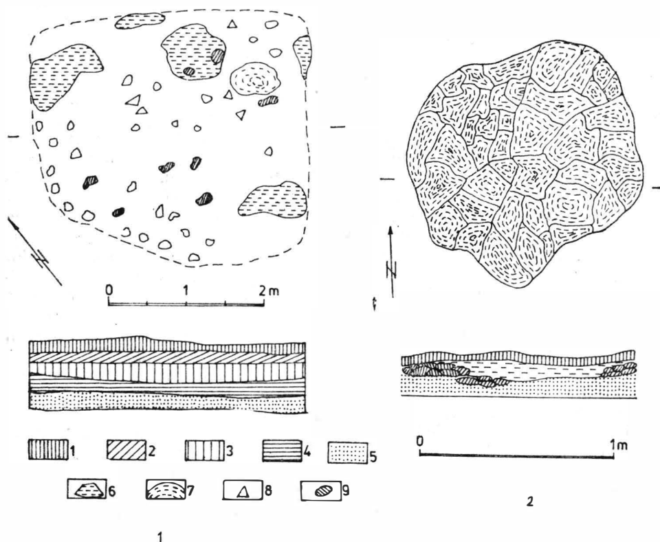
Fig. 9. Botoșana, jud. Suceava. Planul și profilul locuinței 14 (1) și al vetrei 1 (2); 1 sol arabil; 2 nivel prefeudal; 3 nivel și locuință de epocă Latène; 4 sol brun închis; 5 sol viu; 6 resturi de chirpici; 7 resturi de vatră; 8 fragmente ceramice; 9 pietre.
