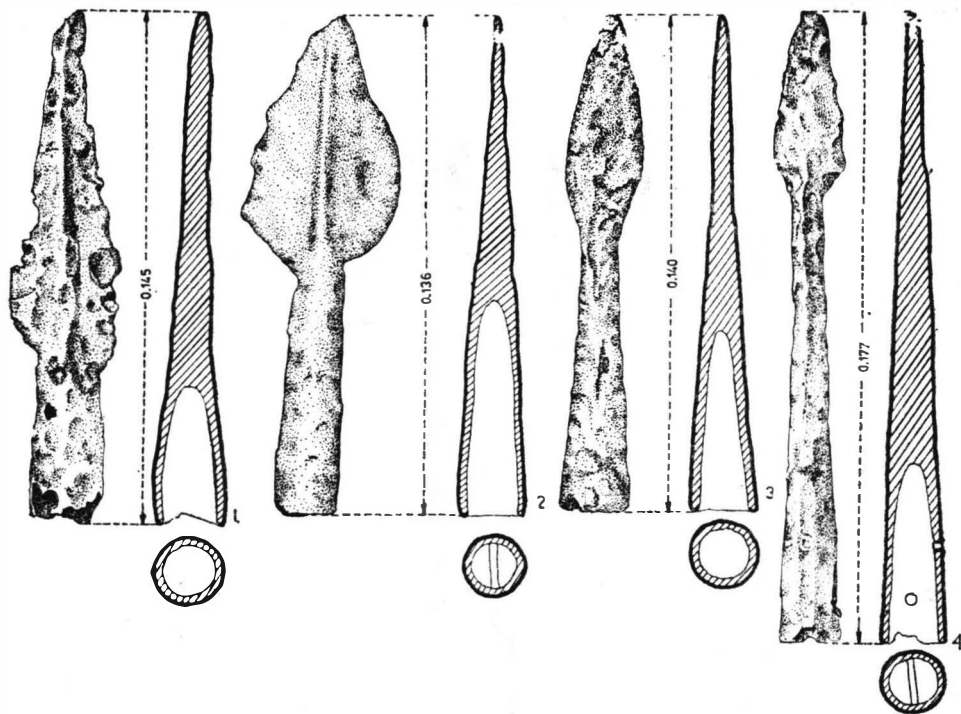
Fig. 11. Botoșana, jud. Suceava. Vîrfuri de lance; 1 locuința 7; 2 semibordeiul 5; 3 locuința 8; 4 din stratul de cultură.
