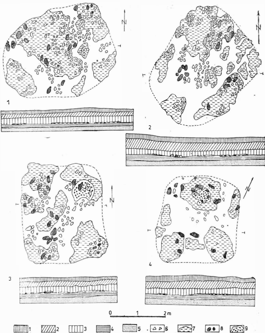
Fig. 8. Botoșana, jud. Suceava. Planul și profilul locuințelor 10, 11, 12, 13; 1 sol arabil; 2 strat prefeudal; 3 nivel și locuințe de epocă Latene; 4 sol brun închis; 5 sol viu; 6 fragmente ceramice; 7 resturi de chirpici și pământ ars; 8 pietre; 9 resturi de vatră.
