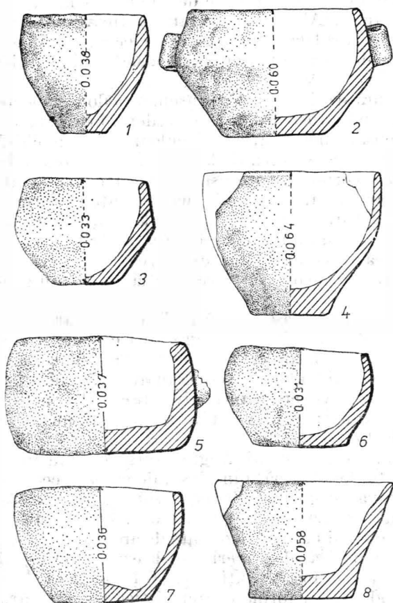
Fig. 15. Botoșana, jud. Suceava. Ceramică lucrată cu mina; 1, 3, 5 semibordeiul 4; 2 locuința 11; 4 locuința 3; 6 locuința 5; 7 semibordeiul 10; 8 din stratul de cultură.
