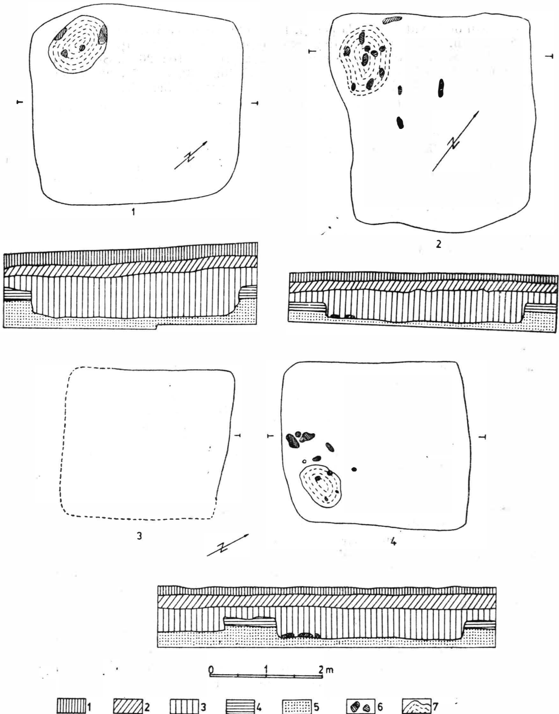
Fig. 3. Botoșana, jud. Suceava. Planul și profilul semibordeiilor 5, 9, 6, 7; 1 sol arabil; 2 nivel prefeudal; 3 nivel și semibordeie de epocă Latène; 4 strat de culoare brun închisă; 5 sol viu; 6 pietre; 7 resturi de vatră.
