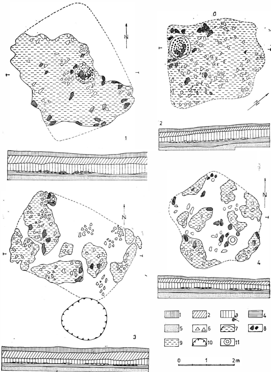
Fig. 6. Botoșana, jud. Suceava ; Planul și profilul locuințelor 2, 3, 4, 5; 1 sol arabil; 2 nivel prefeudal; 3 nivel și locuințe de epocă Latène; 4 sol brun închis; 5 sol viu; 6 fragmente ceramice; 7 resturi de vatră; 8 pietre; 9 pământ ars și chirpici; 10 groapă; 11 vas întreg.
