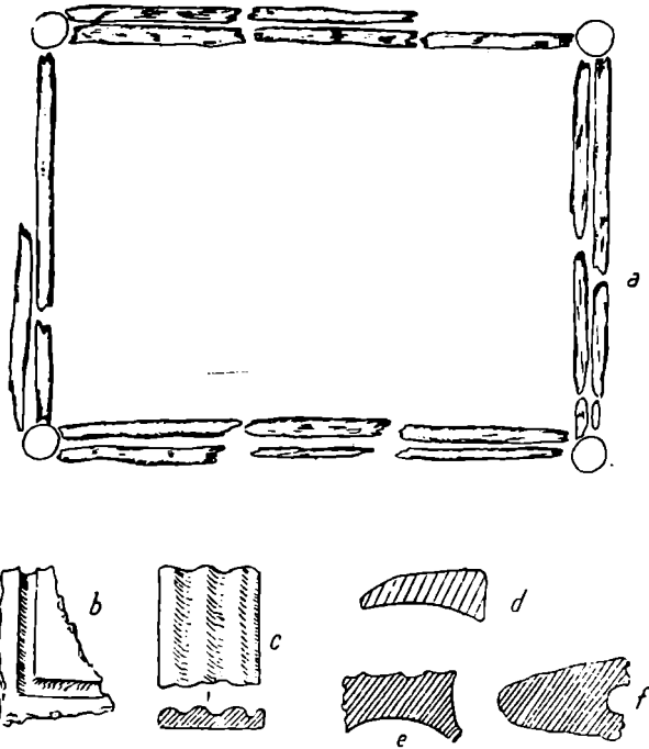
Fig. 4. — Terchești—Chitita. Detalii de construcție de la locuința nr. 1. a, cadru de birne de la baza pereților cu urmele de pari; b—f, bucăți de pereți cu urme de pari și birne.
