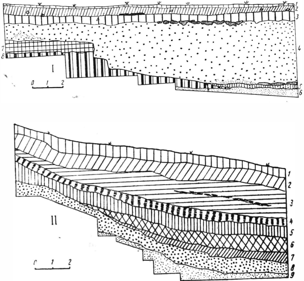
Fig. 3. — I. Profilul peretelui de est al șanțului nr. 2, cu secțiune prin bordeiul nr. 1 și locuința nr. 1 : 1, sol vegetal și humus ; 2, sol brun cu resturile așezării din faza Monteoru Ic 2 ; 3, sol brun-cenușiu cu resturile locuinței de suprafață aparținând nivelului I al fazei Monteoru Ic 3 ; 4, sol brun-cenușiu al nivelului II, cu bordeie aparținând fazei Monteoru Ic 3 ; 5, sol galben-cenușiu cu resturi din faza Monteoru Ic 4 ; 6, sol galben-nisipos ; 7, sol brun-gălbui ; 8, sol galben clisos. II. Profilul peretelui de vest al șanțului nr. 5 : 1, sol arat și cu humus ; 2, sol cenușiu cu resturile așezării din faza Monteoru I Ib ; 3, sol negru-cenușiu cu urmele locuințelor din faza Monteoru IIa ; 4, sol brun-negricios aparținând nivelului Monteoru Ia ; 5, sol cenușiu cu resturile așezării din faza Monteoru Ib ; 6, strat negru cu mult cărbune, aparținând nivelului Monteoru Ic 2 ; 7, sol galben cu cărbune și cenușă, aparținând fazei Monteoru Ic 3 ; 8, sol galben clisos ; 9, sol galben nisipos.
