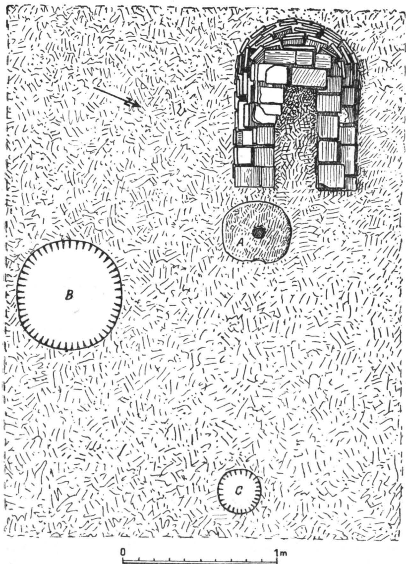
Fig. 13. — Cernica. Planul atelierului-bordel cu cuptor din secțiunea XX—XXI; A, piatră de rîșniță, găsită în dreptul gurii cuptorului; B, groapă pentru cărbune; C, groapa de par, care susținea acoperișul de lemn.
