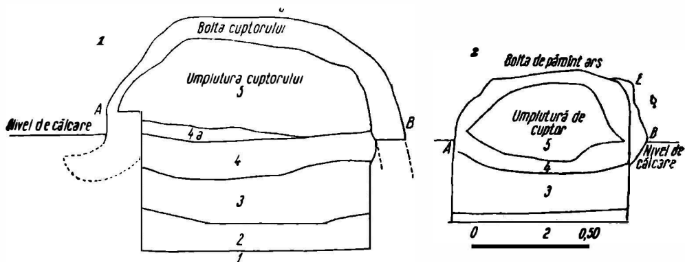
Fig. 10. — Cernica. 1, 2, profilele unor secțiuni prin cuptoarele de pline ale bordeielor feudale nr. 3 și 4. 1, argilă vineție-gălbuie, cu concreții calcaroase; 2, loess galben cu concreții; 3, loess castaniu; 4, pământ ars de la fundul cuptorului; 4 a, lentilă conținând cenușe, cărbuni, pământ ars; 5, umplutura cuptorului compusă din pământ negru și cenușiu conținând bucăți de chirpici, cărbuni, pietricele, pământ ars.
