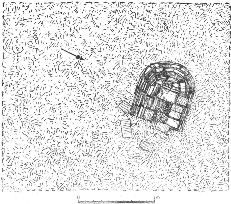
Fig. 12. — Cernica. Planul atelierului-bordei cu cuptor din secțiunea XVII.
