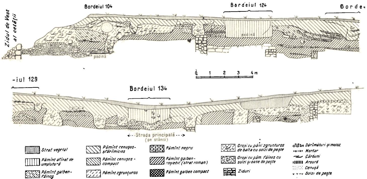
Fig. 14. — Profilul malului de nord-vest al sectorului C.
