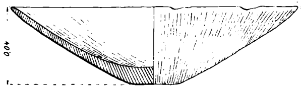
Fig. 1. — Vasul de piatră descoperit pe Grădiștea Ulmilor.
