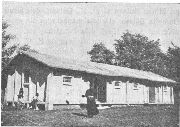
Magazinul de bucate dela Răsmirești absolut tot de beton armat.
