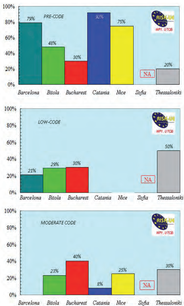
Figura 3. Caracterizarea fondului imobiliar construit, în procente, în funcție de tipul de cod antiseismic în vigoare la data construcției după FEMA / HAZUS: fără cod, cod inferior, cod moderat. RISK UE Project
