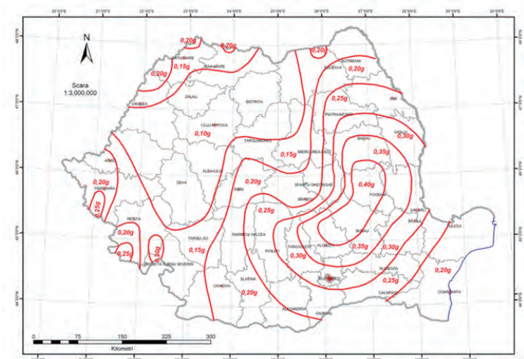
Figura 17. P100-1/2013, Harta de zonare a hazardului seismic
