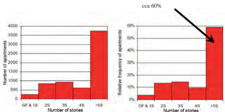
Figura 21. București. Clădiri din clasa 1 de risc seismic grupate în funcție de nivelul de înălțime
