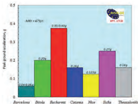
Figura 2 (a). Hazardul seismic: accelerația seismică maximă pentru proiectarea construcțiilor având 50 ani și, respectiv, 475 ani interval mediu de recurență.
