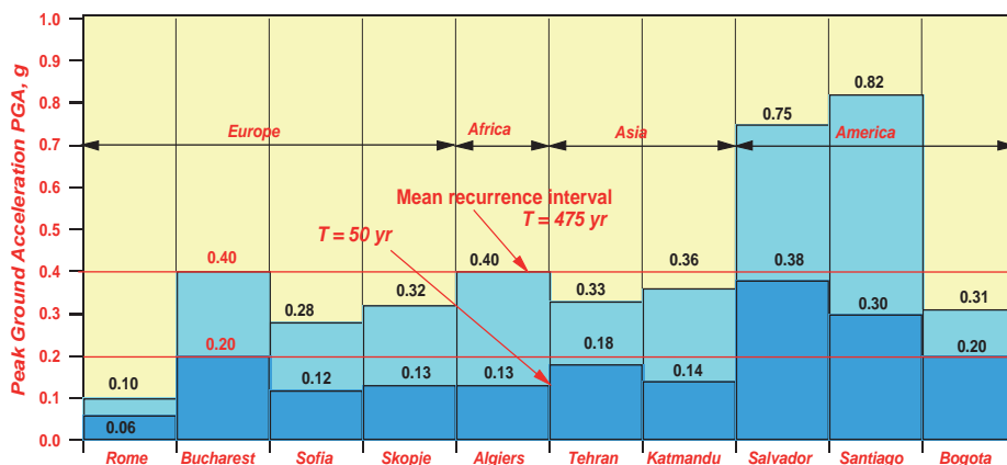
Figura 1 (a). Hazardul seismic: accelerația seismică maximă pentru proiectarea construcțiilor având 50 ani și, respectiv, 475 ani interval mediu de recurență. U.N. RADIUS Project
