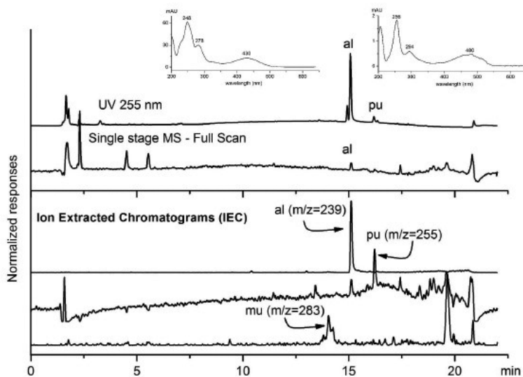
Fig. 5. Imagine care susține identificarea coloranților din roibă ( Rubia tinctorum , madder) în zona inferioară sprang a căței 7491T din colecția Muzeului de Etnografie Brașov. Analiză efectuată prin LC-DAD-MS (vezi text).
