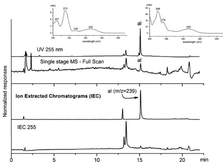
Fig. 6. Imagine care susține identificarea alizarinei sintetice (1871) în intervenții anterioare efectuate asupra căței 7491T din colecția Muzeului de Etnografie Brașov. Analiză efectuată prin LC-DAD-MS (vezi text).
