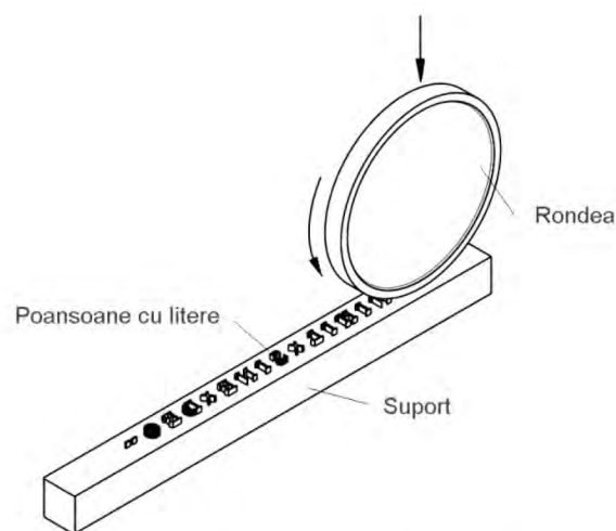
Fig. 4. Imprimarea cantului rondulei cu deviza incusă.
