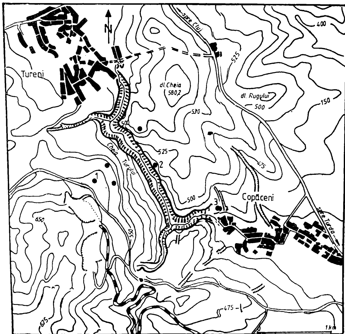
Figura 2 — Situația topografică a celor mai importante descoperiri aparținând bronzului timpuriu din Cheile Turenilor. 1. Tureni — „La Furci”; 2. Tureni — „Poderei”; 3. Copăceni — „La Moară”.
